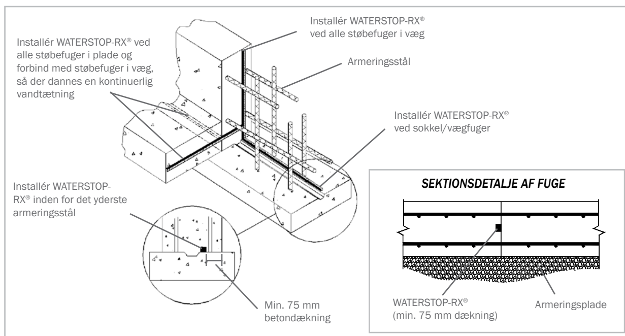
Typisk fundamentdetaljer af WATERSTOP-RX®
