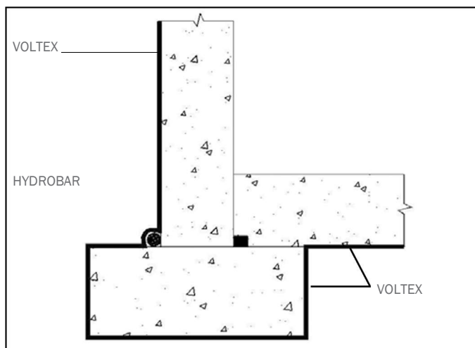
Installér HYDROBAR® direkte i det indvendige hjørne i overgangen mellem sokkel og væg
