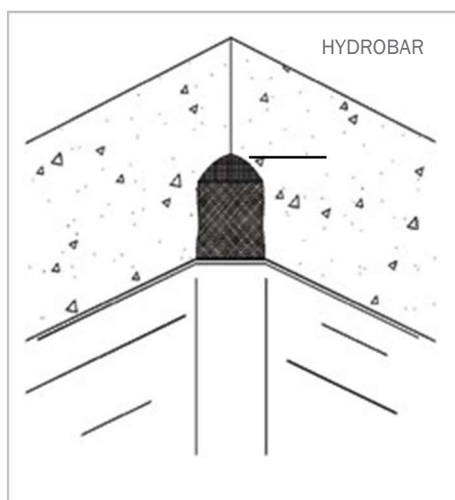
Fundamentvæg Udvendige Indvendige hjørner
