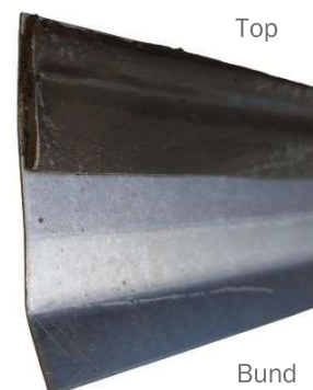
Aktiv bentonit tætningsliste
