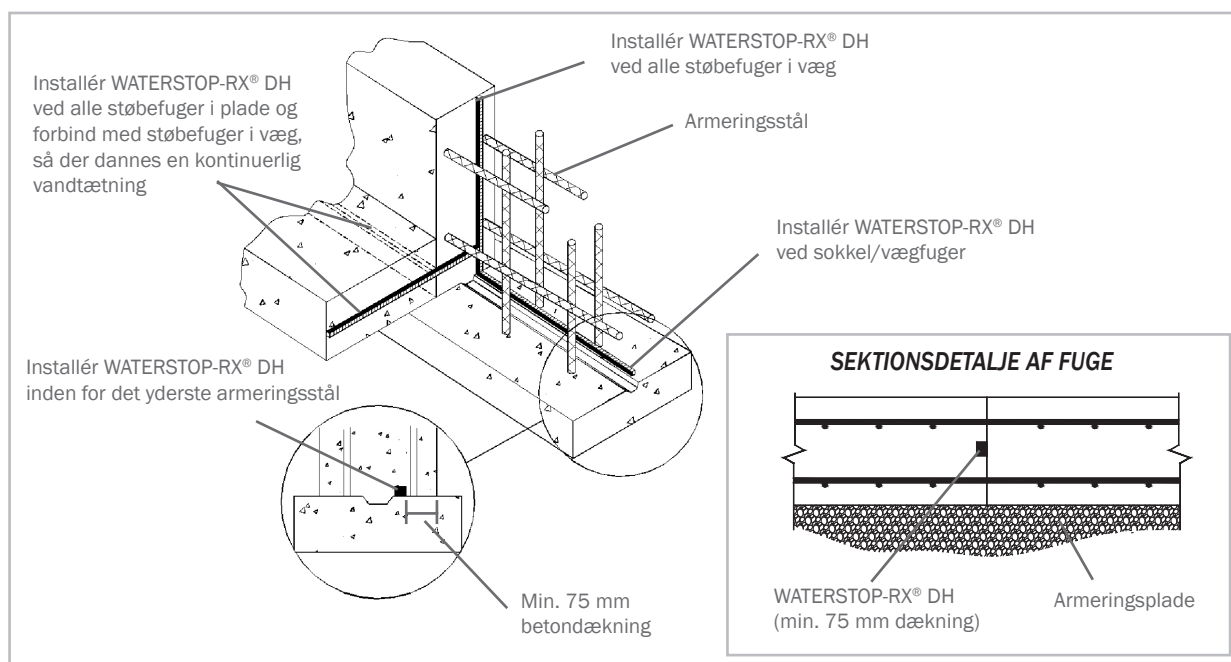
Typisk fundamentdetaljer af WATERSTOP-RX® DH
